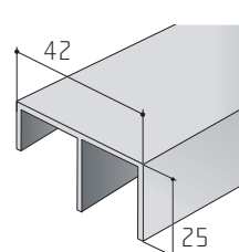
Dolní vodící profil S30/45
