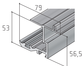
S45 - Horní profil
