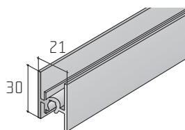
Příčka S65
