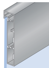
Rámový profil S45-100
