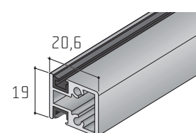
Příčka pro profily A a B
